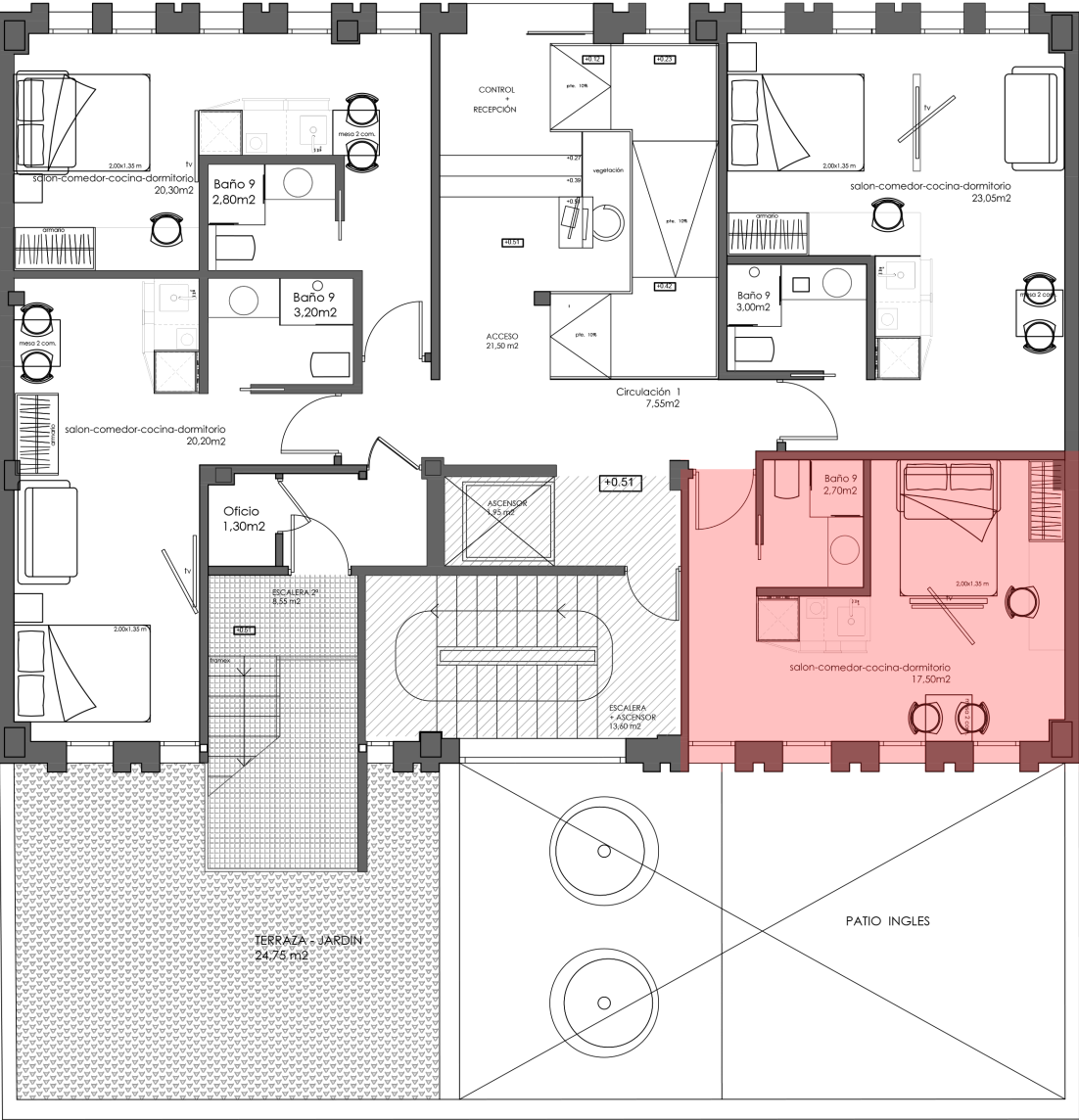
CALLE ROMA N°16+18 _ PLANTA BAJA 0 1 2 3 4 5 Sup. Construida = 161,45 m² Sup. Util = 144,75 m² + 24,75 terraza
