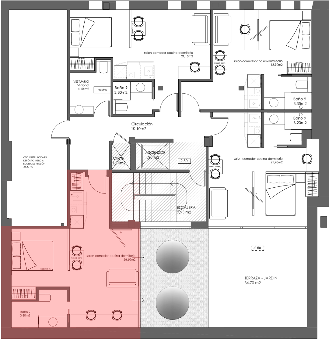
CALLE ROMA Nº16+18 _ PLANTA SOTANO 0 1 2 3 4 5 Sup. Construida = 228,95 m 2 Sup. Util = 192,90 m 2
