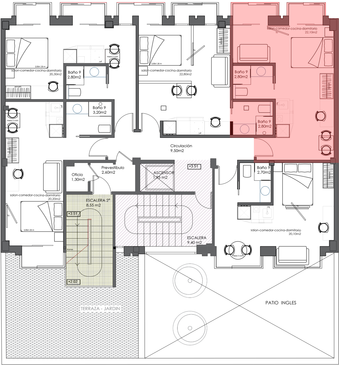
CALLE ROMA N°16+18 _ PLANTA PRIMERA 0 1 2 3 4 5 Sup. Construida = 173,90 m 2 Sup. Util = 150,90 m 2
