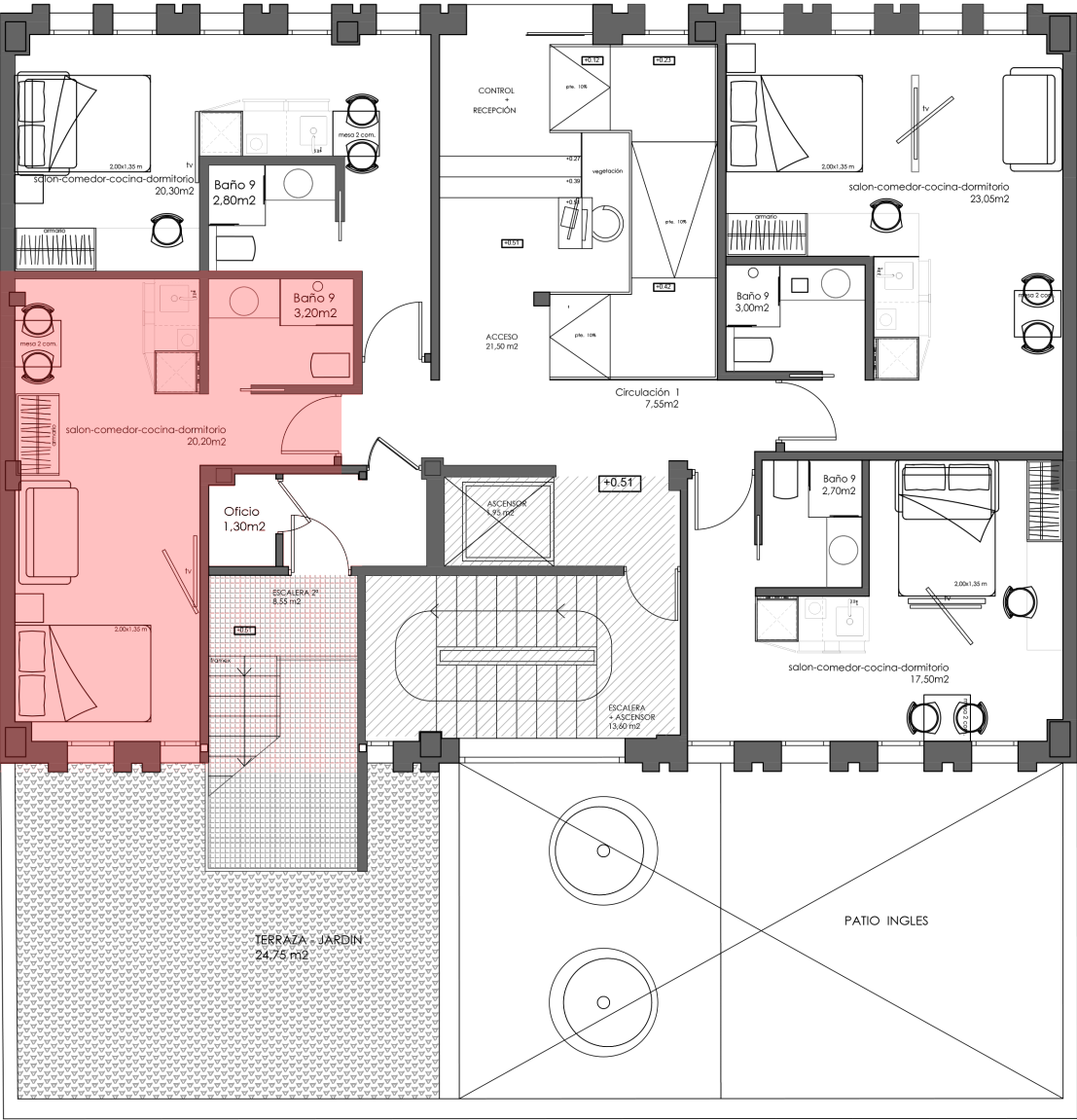
CALLE ROMA Nº16+18 _ PLANTA BAJA 0 1 2 3 4 5 Sup. Construida = 161,45 m2 Sup. Util = 144,75 m2 + 24,75 terraza
