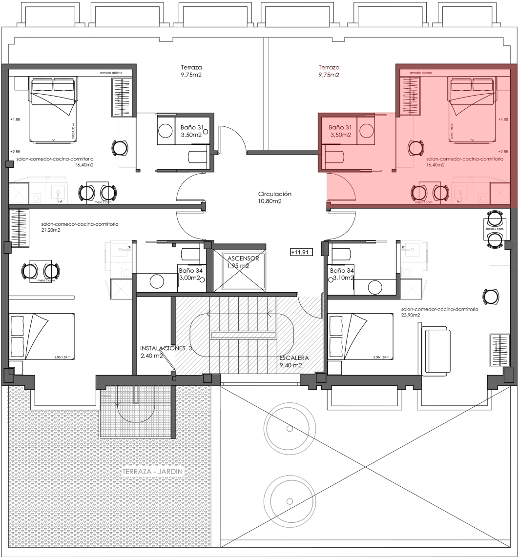
CALLE ROMA N°16+18 _ PLANTA CUARTA 0 1 2 3 4 5 Sup. Construida = 161,80 m2 Sup. Util = 111,05 m2
