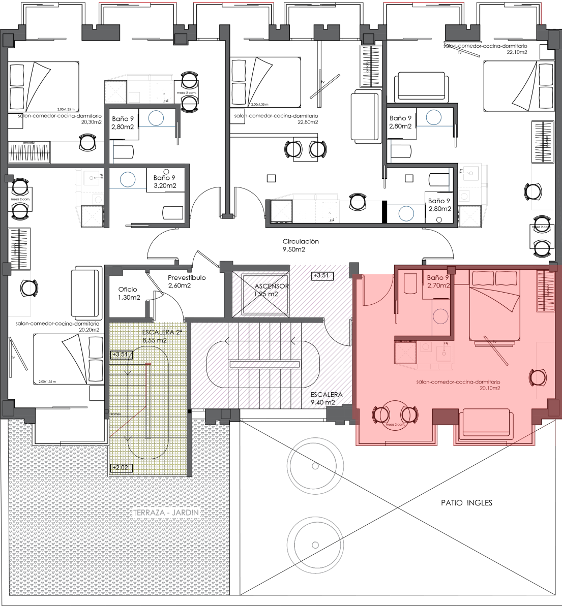
CALLE ROMA N°16+18 _ PLANTA PRIMERA 0 1 2 3 4 5 Sup. Construida = 173,90 m² Sup. Util = 150,90 m²
