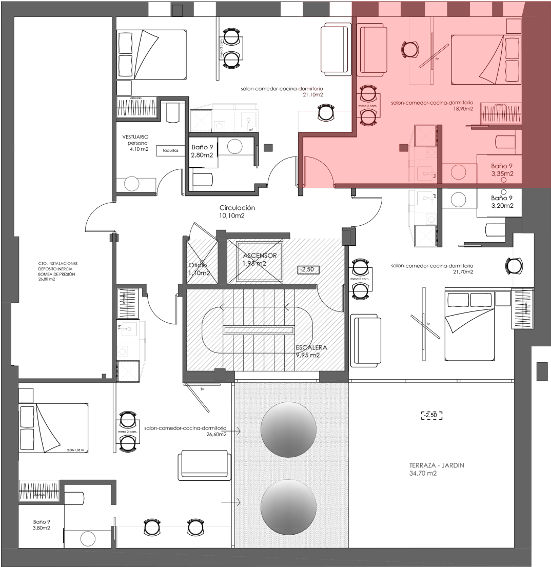
CALLE ROMA N°16+18 _ PLANTA SOTANO 0 1 2 3 4 5 Sup. Construida = 228,95 m 2 Sup. Util = 192,90 m 2
